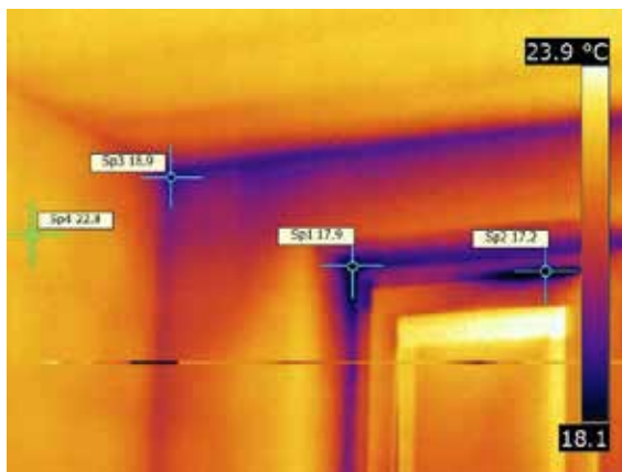
Obraz widziany kamerą termowizyjną (okno)
