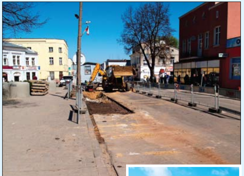
Usuwanie starej nawierzchni z ul. Warszawskiej
